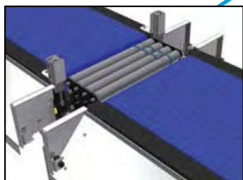
TRANSFERENCIA CON RODILLO ACTIVO
