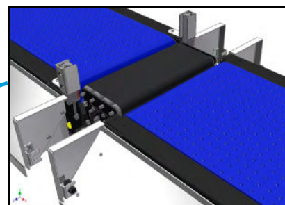
TRANSFERENCIA CON RODILLO RECUBIERTO ACTIVO
